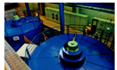
Casa de máquinas de la planta hidroeléctrica Cariblanco. ARCHIVO
